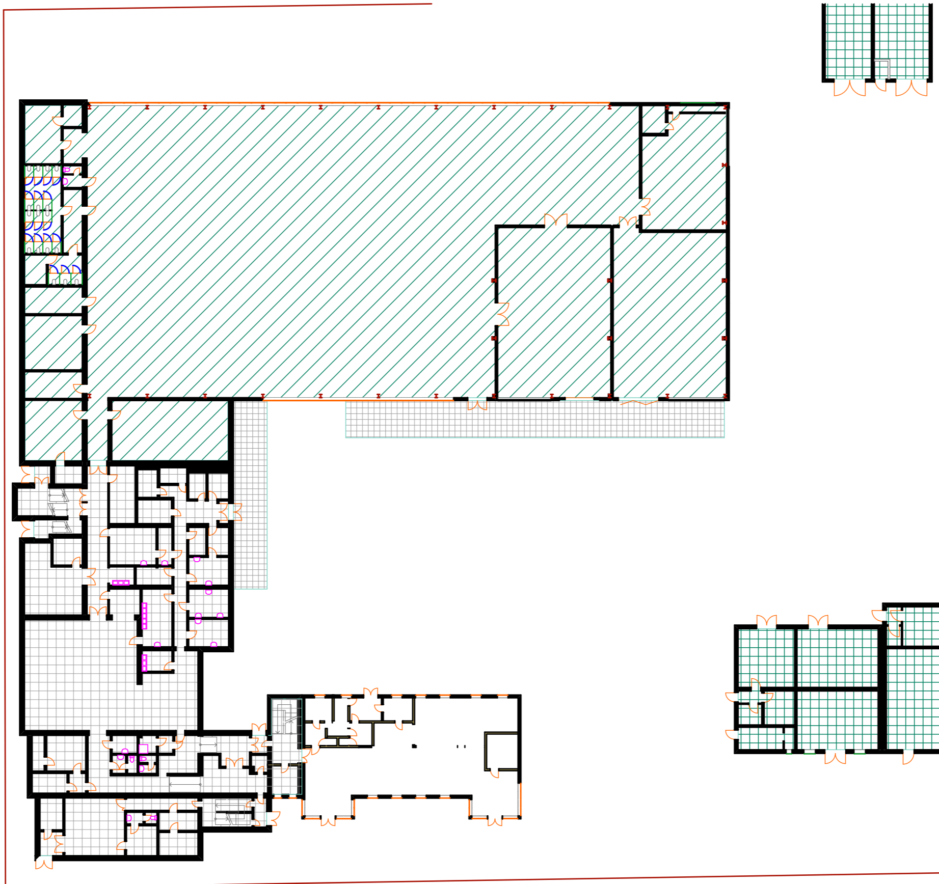
KIVI 2 KVARTALIKINNISTU TOOTMISPLOKI PÕHIKORRUSE PLAAN M1:400
